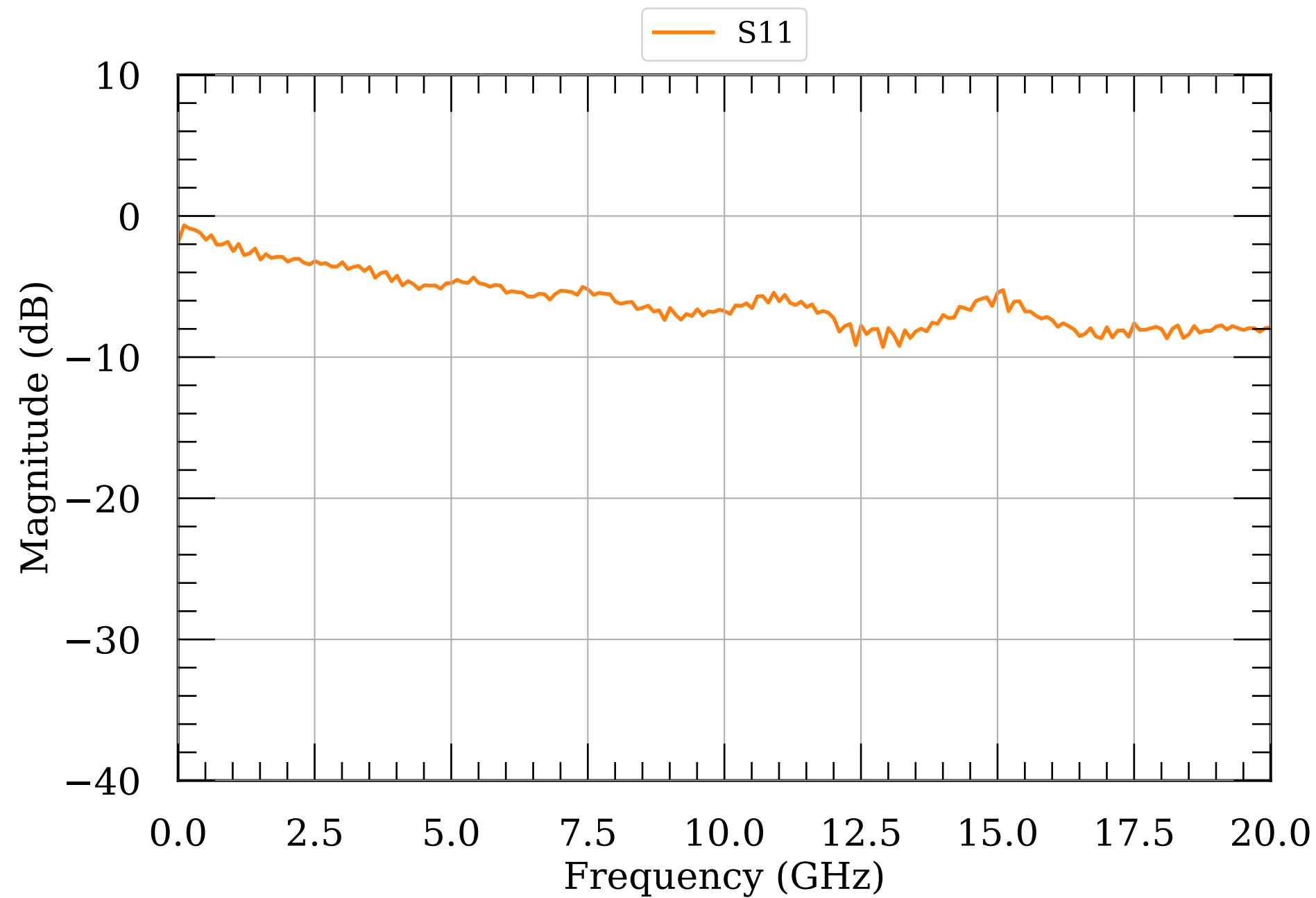
LNA S-params module083
